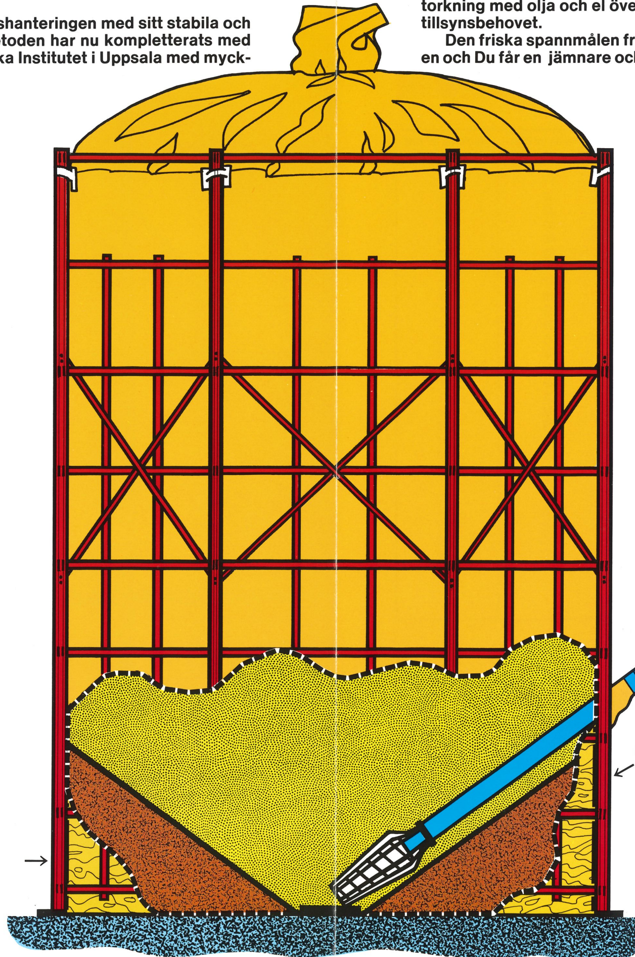
SAMLE LUFTTÄT med konisk botten monterad ovan golv. Tömningsskruv med lufttät lucka. Skruvuttag i sidan. 6 mm vattenfast plywood på sidorna. 500 mm Ø plywood till skydd för skruv i botten.
