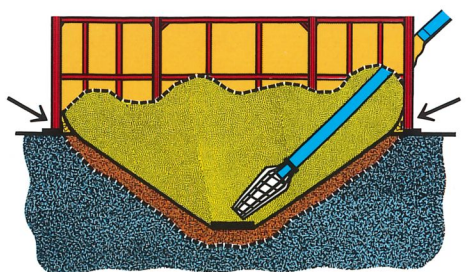
Konisk botten helt nersänkt under golv för ytterligare volym.
